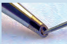
3. Lötspitze mit Lot füllen
